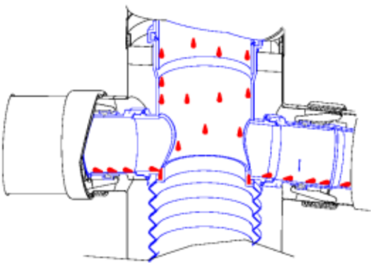
Figure 1 – Evacuation des condensats sur té de piquage
