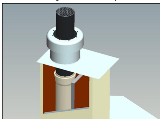
Figure 8b – Terminal Configuration Réutilisation d'un conduit existant
