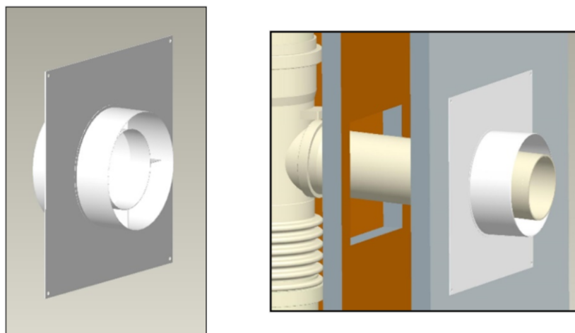
Figure 7 – Plaque de finition avec élément de centrage (gauche) et Conduit de liaison (droite) Configuration Réutilisation d'un conduit existant
