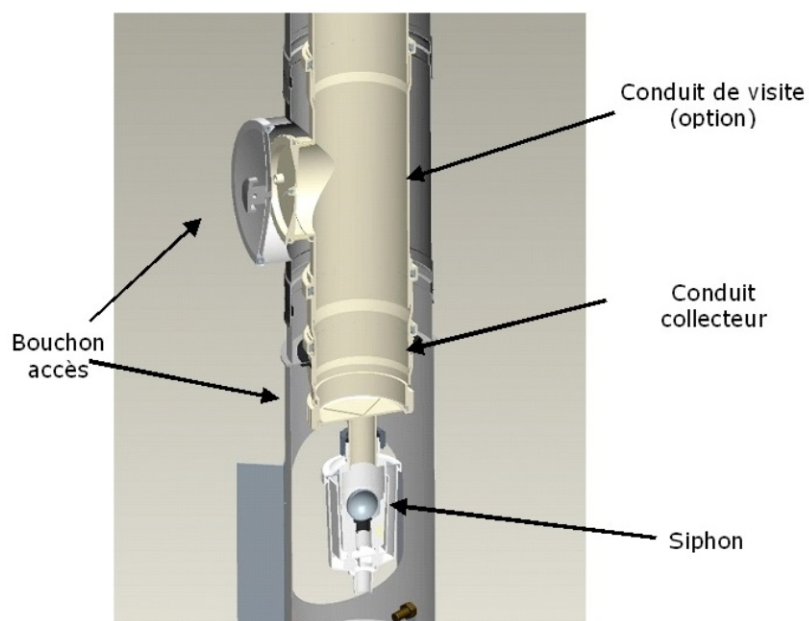
Figure 4 – Conduit de visite et bas de colonne Configuration concentrique
