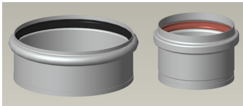
Figure 13 – Dispositif d'obturation et de maintenance du conduit de liaison composé d'un bouchon de sécurité pour l'évacuation des produits de combustion et d'un bouchon de sécurité pour l'amenée d'air comburant
