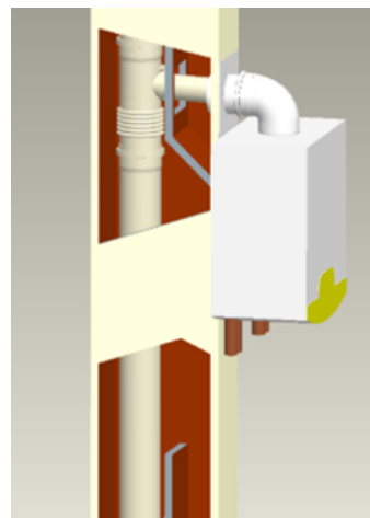
Figure 12c – Connexion étage
