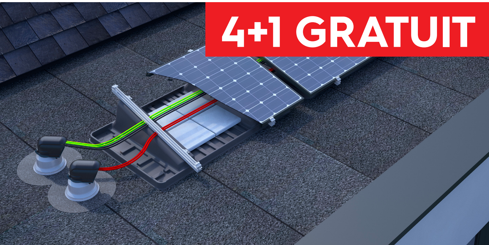
Passage de toiture Multivent
