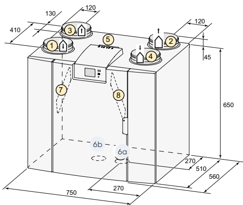
4-0 aansluitingen
