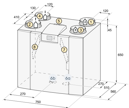
4-0 aansluitingen
